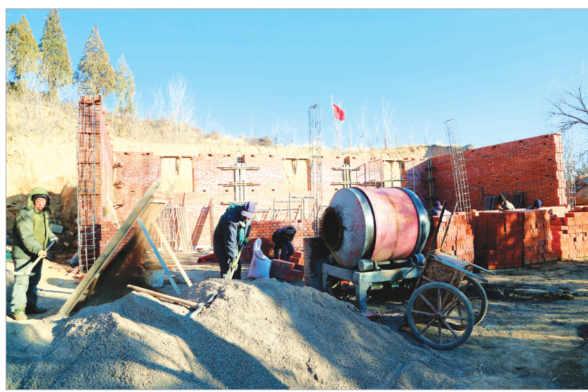
郊区桃林沟村优化供水系统项目水源取自北环路魏家峪桥西侧的市政自来水管网，主要建设一座一级泵站和一座二级泵站，均为单层砖混结构。图为日前拍摄的项目建设现场。杨园园摄
